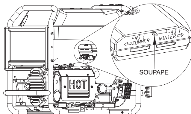
Figure 9 - Soupape d'été/hiver
