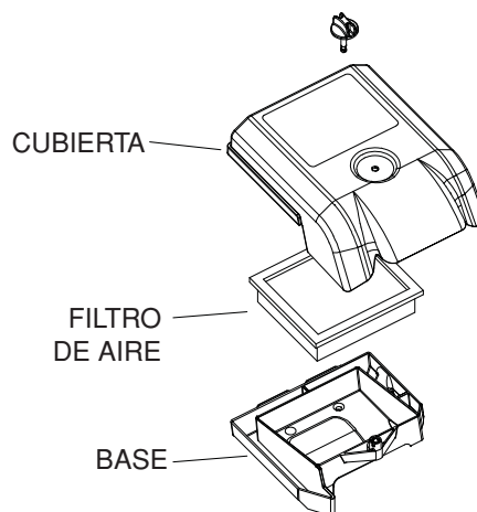
Figura 24 - Filtro de aire de 10kW (Nº de parte 073111)
