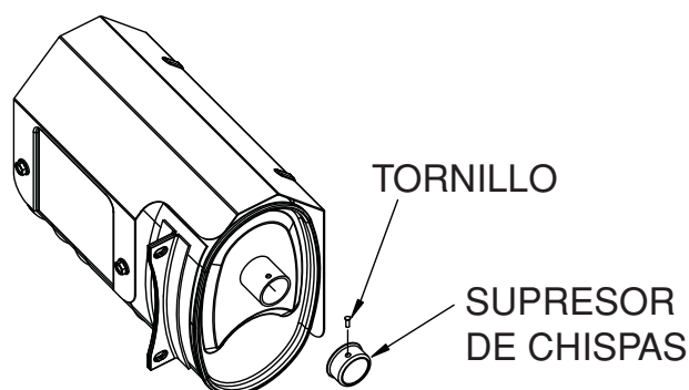
Figura 26 - Supresor de chispas de 6.5, 8 y 10kW
