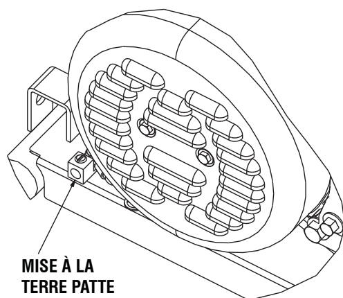
Figure 16 - Mise à la terre de la génératrice
