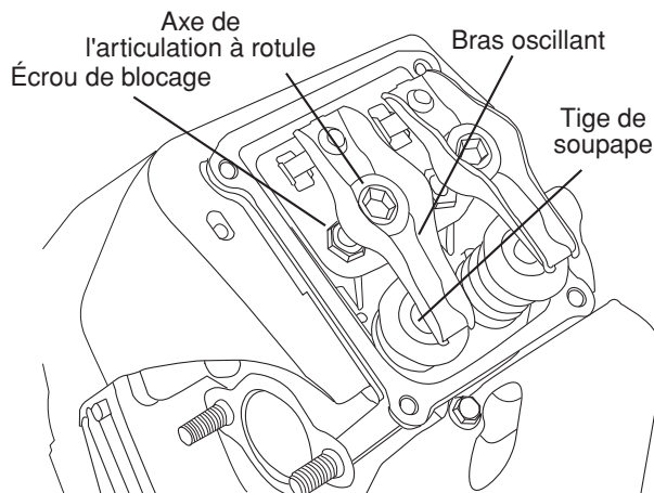
Figure 27 - Réglage du jeu des soupapes
