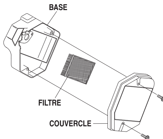
Figure 24 - Filtre à air, 10 kW (N° de pièce 073111)
