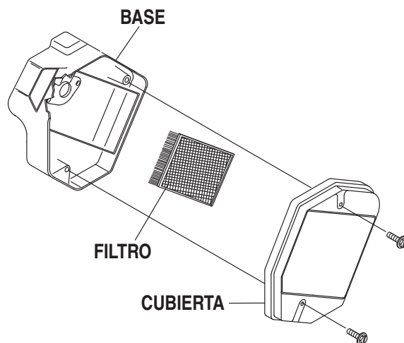
Figura 24 - Filtro de aire de 10kW (Nº de parte 073111)
