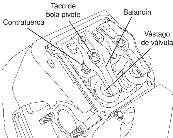
Figura 27 - Ajuste del espacio de la válvula
