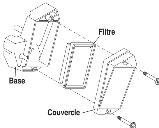
Figure 23 - Filtre à air, 6,5 et 8 kW (N° de pièce 073111)
