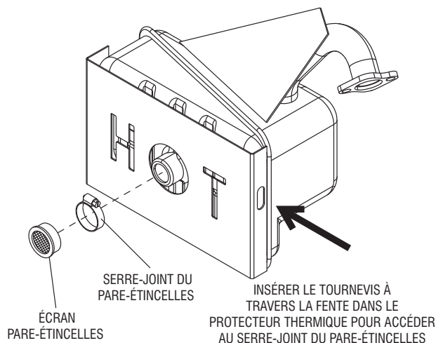
Figure 25 - Pare étincelles, 3,6 kW
