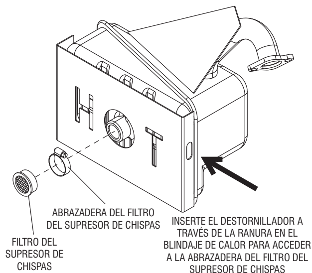
Figura 25 - Supresor de chispas de 3.6kW
