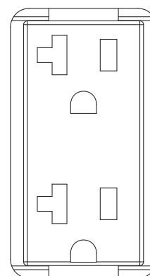
Figura 11 - Receptáculo doble de 120 Volt AC, 20 amperios
