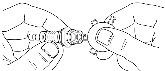
Figura 21 - Espaciamento de la bujía
