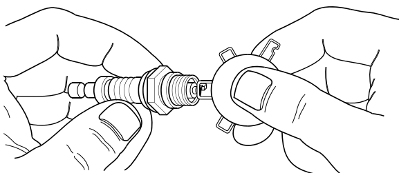
Figure 21 - Écartement de la bougie d'allumage
