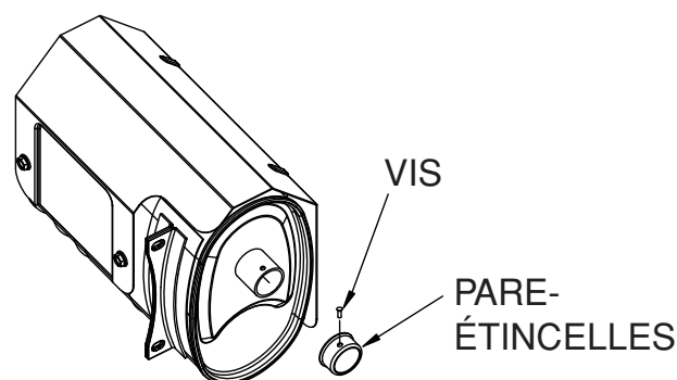
Figure 26 - Pare étincelles, 6,5, 8 et 10 kW
