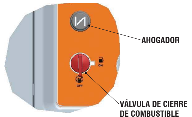
Figura 19 - Válvula de corte de combustible
