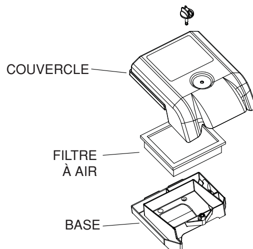
Figure 24 - Filtre à air, 10 kW (N° de pièce 073111)
