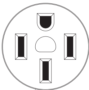
Figura 13 - Receptáculo de 120/240 VAC, 50 amperios
