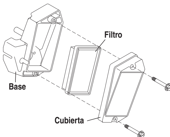
Figura 23 -Filtro de aire de 6.5 y 8kW (Nº de parte 073111)
